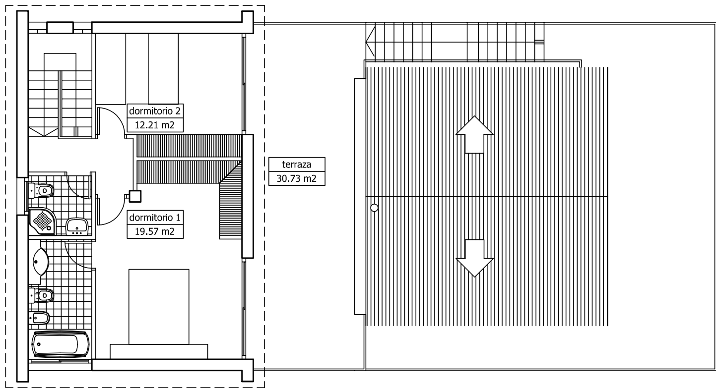
planta alta
